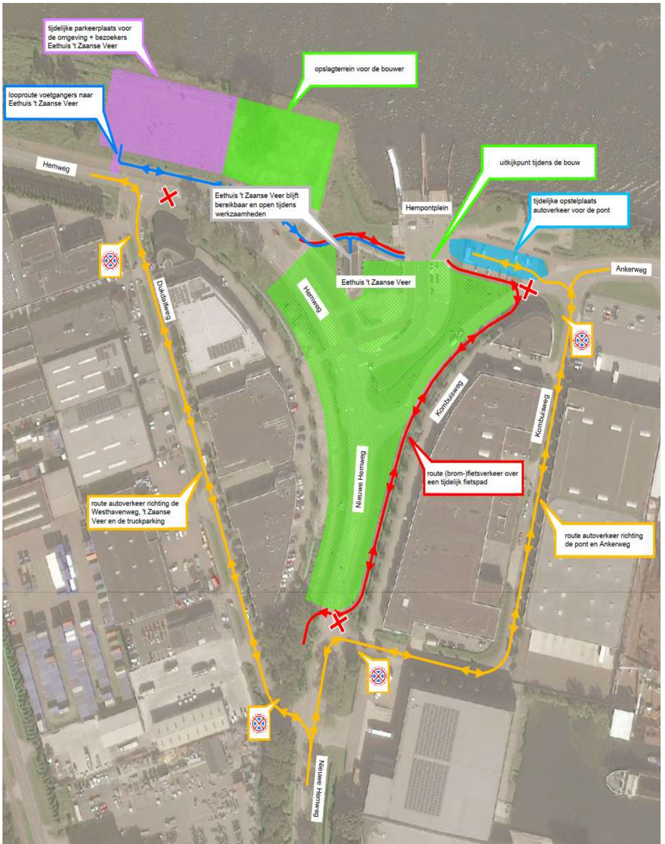
Afbeelding 2: weergave verkeersstromen bouwfase
